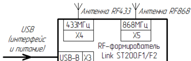
Рисунок Б.4 – Подключение формирователя Link ST200.F1/F2 и Link ST200.F1/F2 «прямой опрос» ВЛСТ 339.04.000-00
